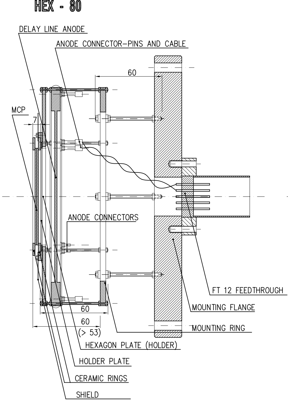
SECTION A-A
