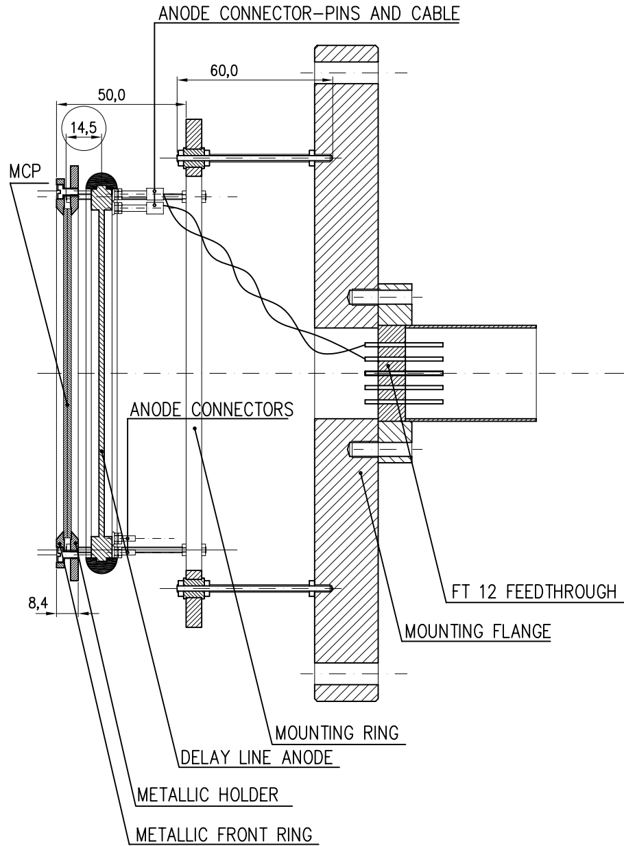
SECTION A-A
